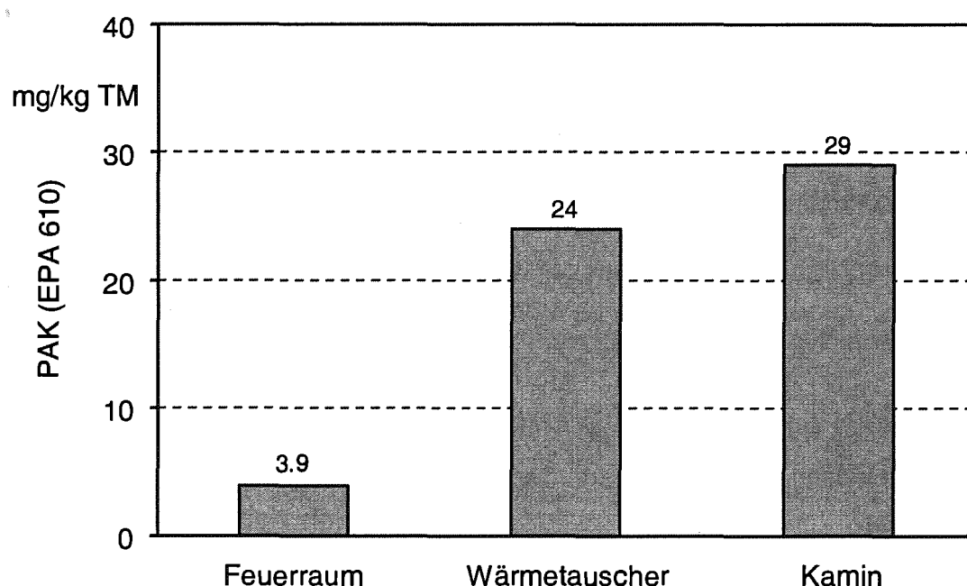
Abb. 31: PAK-Gehalte von Aschen aus verschiedenen Abscheidungsorten des untersuchten Stückholzkessels. - Brennstoff: Buchenscheitholz, Heizleistung: Nennwärmeleistung (Ergebnisse eines einzelnen Verbrennungsversuches).
