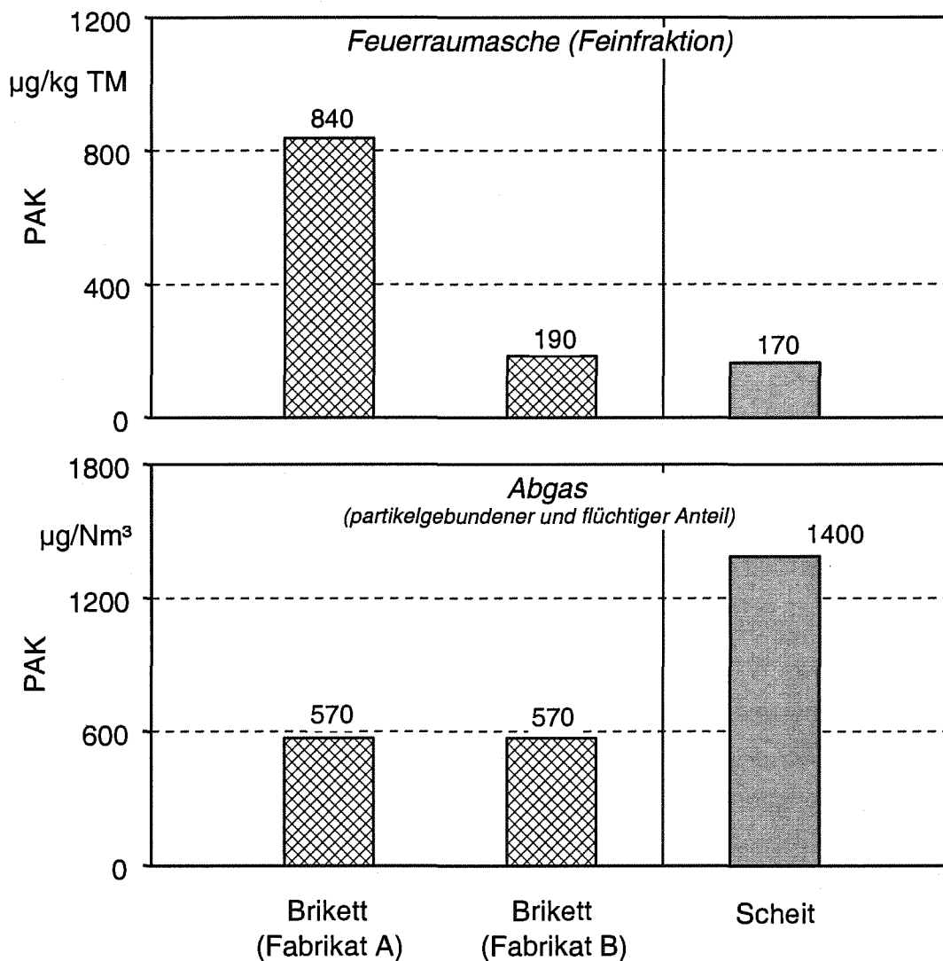
Abb. 42: PAK-Gehalt im Abgas und in der Feuertemasche bei unterschiedlichen Aufbereitungsformen des Brennstoffs. - Dargestellt sind Mittelwerte aus zwei bis vier Versuchen; Heizlast: 70 - 110 %; Brennstoff: Nadelholz; PAK angegeben als Summenwerte nach EPA (Angaben der Abgaskonzentrationen ohne Naphthalin).
