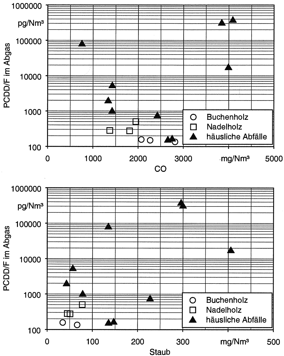
Abb. 48: PCDD/F-Emissionen in Abhängigkeit von CO- und Staubemissionen bei der Verbrennung von naturbelassenem Holz und Mitverbrennung von häuslichen Abfällen. - Feuerungsanlage: "optimierter" Kachelofen; Emissionswerte bezogen auf 13 Vol.-% O 2 .
