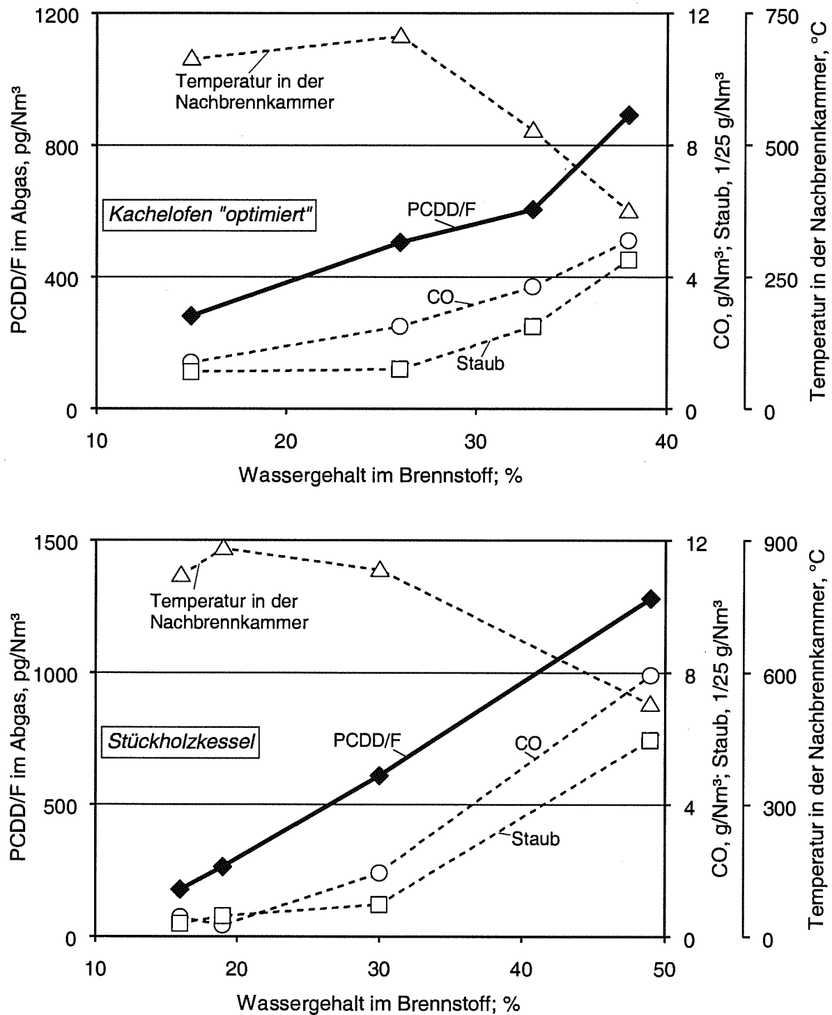
Abb. 44: Abhängigkeit der PCDD/F-Emissionen sowie der Verbrennungsqualität und -temperatur vom Brennstoffwassergehalt. - Brennstoff: Fichtenscheitholz.; Emissionswerte bezogen auf 13 Vol.-% O 2 .
