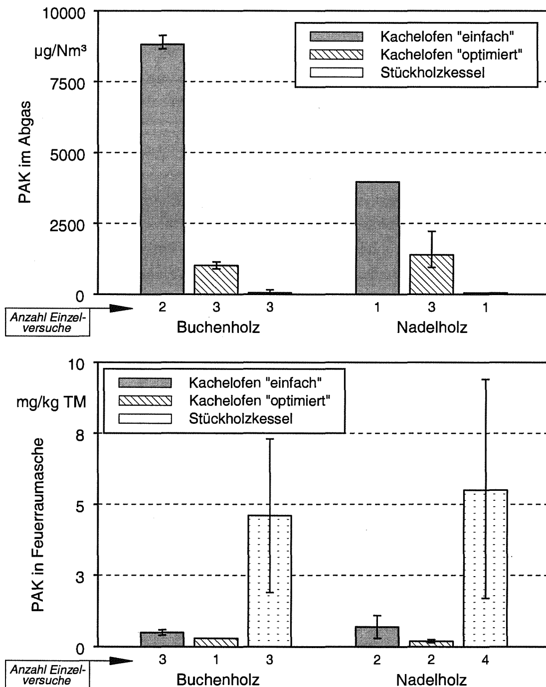
Abb. 40: PAK-Gehalte in Abgas und Feuerraumasche von Verbrennungsversuchen mit Hart- und Weichholz. - Heizlast: 70 - 110 %; Emissionswerte bezogen auf 13 Vol.-% \text{O}_2 ; PAK angegeben als Summenwerte nach EPA ohne Naphthalin.
