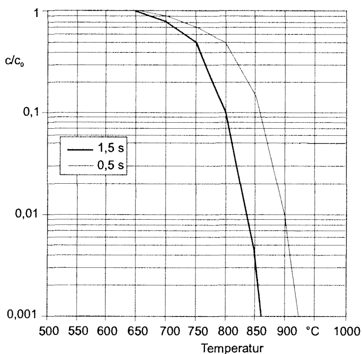
Abb. 6: Thermische Zersetzung von 1,2,3,4-Cl 4 DD in Luft bei Verweilzeiten von 0,5 und 1,5 Sekunden bei verschiedenen Temperaturen ( c/c_0 = relative Konzentration) [57].
