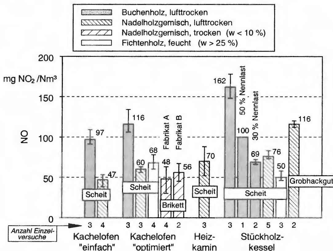
Abb. 24: \text{NO} -Emissionen der untersuchten Hausbrandfeuerungen. - Heizlast bei Einzelfeuerstätten: 70 - 110 %, Heizlast beim Stückholzkessel: ca. 100 % sowie zwei Versuche im Teillastbetrieb; Emissionswerte bezogen auf 13 Vol.-% \text{O}_2 .
