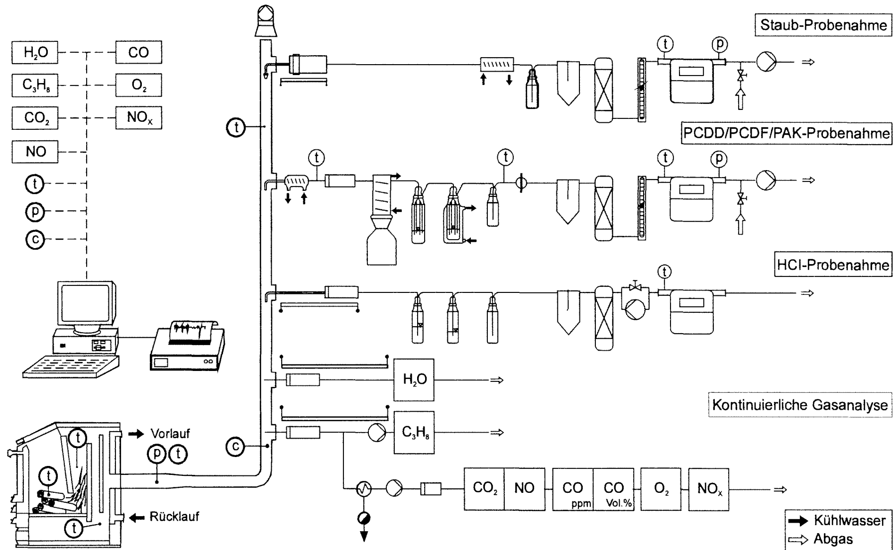
Abb. 11: Schematische Darstellung des Meßgeräteaufbaus im Feuerungsprüfstand.
