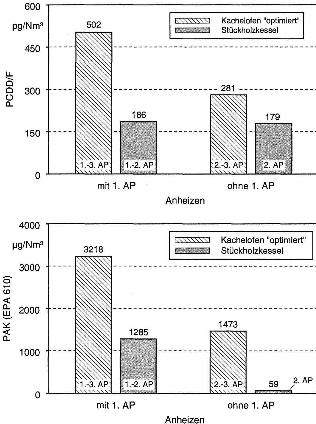
Abb. 37: PCDD/F- und PAK-Emissionen in Abhängigkeit vom Betriebszustand der Feuerungsanlage. - Gegenübergestellt sind Mittelwerte aus Verbrennungsversuchen "mit" und "ohne" die erste Abbrandperiode (AP); Heizlast im betriebswarmen Zustand: ca. 100 %; Brennstoff: lufttrockenes Nadelstehholz.
