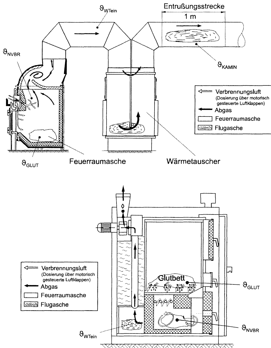
Abb. 16: Darstellung der Entaschungsbereiche und Temperaturmeßstellen.
