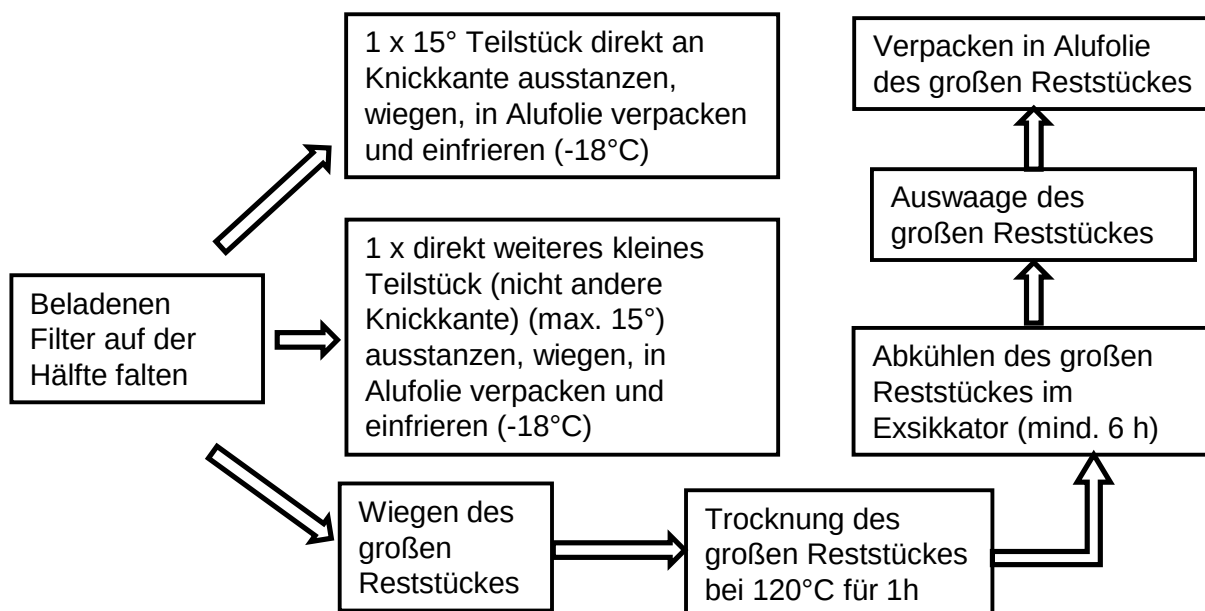
Abbildung 15: Behandlung der großen Planfilter (150 mm) für die Bereitstellung zur stofflichen Analyse
