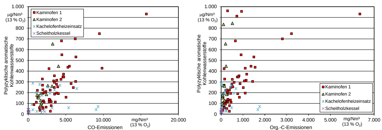
Abbildung 96: Partikelgebundene Emissionen an polyzyklischen aromatischen Kohlenwasserstoffen (PAK) in Abhängigkeit vom Kohlenmonoxidausstoß und org.-C-Emissionen
