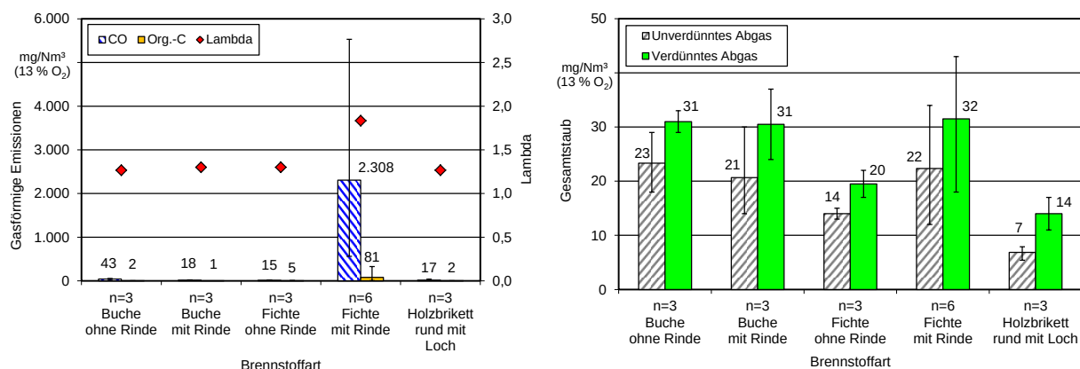
Abbildung 77: Einfluss der Holzart und des Aschegehaltes auf die gasförmigen Emissionen und Staubemissionen im unverdünnten und verdünnten Abgas. Feuerung: Scheitholzkessel HDG Navora, Brennstoffe: Buche und Fichte mit und ohne Rinde sowie ein rundes Holzbrikett mit Loch, Durchmesser des Scheitholzes: 10-12 cm (n = Anzahl der Messungen)
