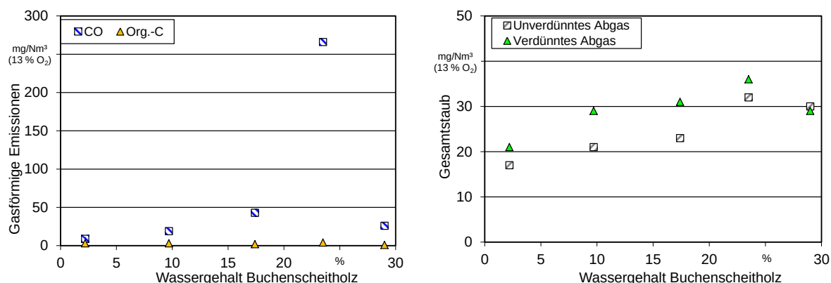
Abbildung 81: Einfluss des Wassergehaltes bei Buchenscheitholz auf die gasförmigen Emissionen und Staubemissionen im unverdünnten und verdünnten Abgas. Feuerung: Scheitholzkessel HDG Navora, Brennstoff: Buche ohne Rinde mit D10 - D12
