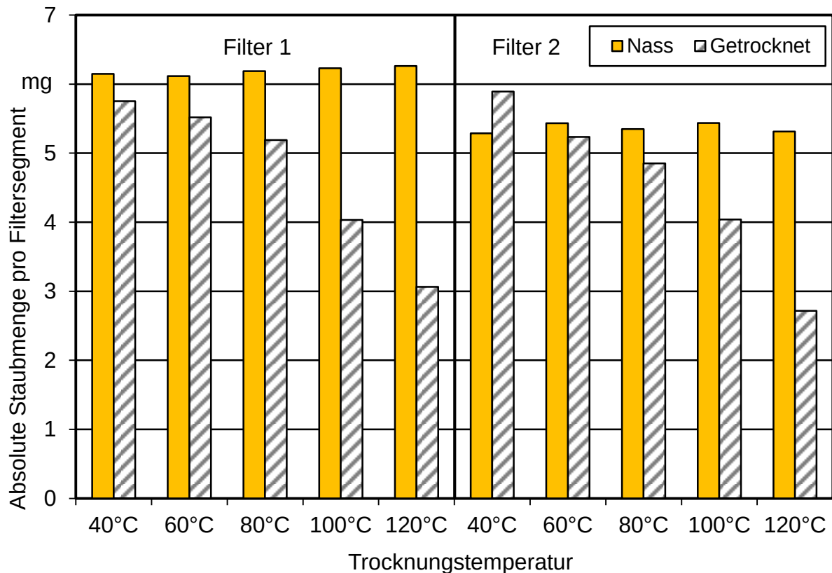
Abbildung 31: Staubmasseänderung durch die thermische Filter-Nachbehandlung bei verschiedenen Temperaturen im Vergleich zur unbehandelten Staubbela- dung. Feuerung: Kaminofen 1 Buderus blueline Nr. 12, Brennstoff: Bu- chennormscheit; Probenahme im verdünnten Abgas bei 44°C
