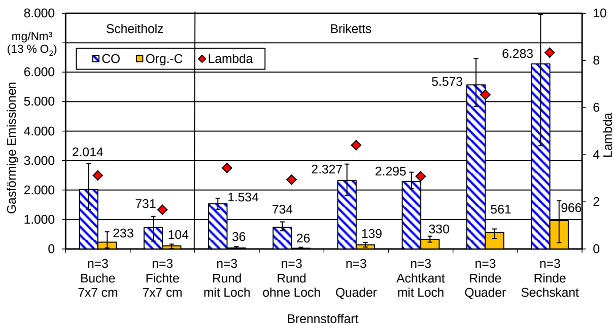
Abbildung 75: Vergleich der gasförmigen Emissionen von Buche- und Fichtennormscheiten mit Holzbriketts und reinen Rindenbriketts. Feuerung: Kachelofenheizung Brunner KKE 33, Nachlegemasse: ca. 2,1 kg ( n = Anzahl der Messungen)
