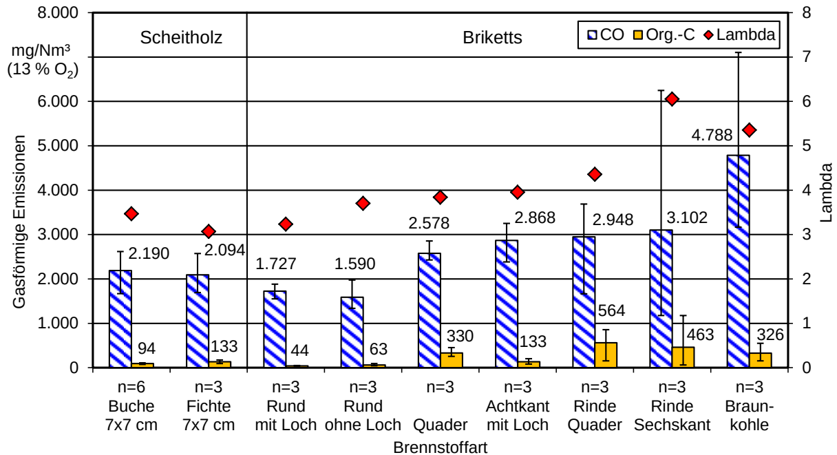
Abbildung 67: Vergleich der gasförmigen Emissionen von Scheitholz mit Holzbriketts, reinen Rindenbriketts und Braunkohlebriketts. Feuerung: Kaminofen 2 Fireplace Santa Fe, Nachlegemenge: ca. 1,6 kg ( n = Anzahl der Messungen).
