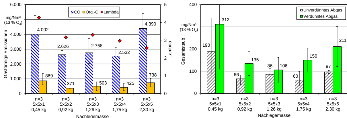
Abbildung 46: Einfluss der Nachlegemenge auf die gasförmigen und staubförmigen Emissionen im unverdünnten und verdünnten Abgas bei einer Kantenlänge von 5 x 5 x 25 cm. Feuerung: Kaminofen 1 Buderus blueline Nr. 12, Brennstoff: Buche ohne Rinde, Wassergehalt: ca. 14,5 %; Anzahl der Scheite (1 bis 5) und somit Brennstoffmasse steigend (n = Anzahl der Messungen)
