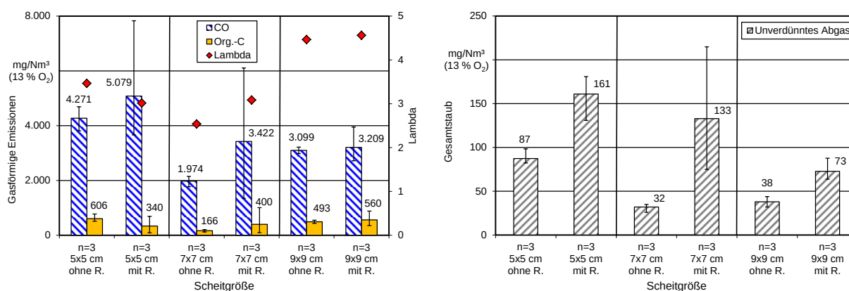
Abbildung 62: Einfluss einer nachrüstbaren Regelung auf die gasförmigen Emissionen sowie Staubemissionen im unverdünnten Abgas bei drei unterschiedlichen Scheitgrößen. Feuerung: Kaminofen 1 Buderus blueline Nr. 12, Brennstoff: Buche ohne Rinde, Auflegemasse: 2,5 kg (n = Anzahl der Messungen)
