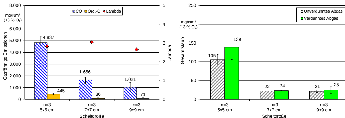
Abbildung 70: Einfluss der Scheitgröße auf die gasförmigen Emissionen und Staubemissionen im unverdünnten und verdünnten Abgas. Feuerung: Kachelofenheizeinsatz Brunner KKE 33, Brennstoff: Buche ohne Rinde, Auflegemasse: 2,4 kg, Wassergehalt: 13,1 % ( n = Anzahl der Messungen)
