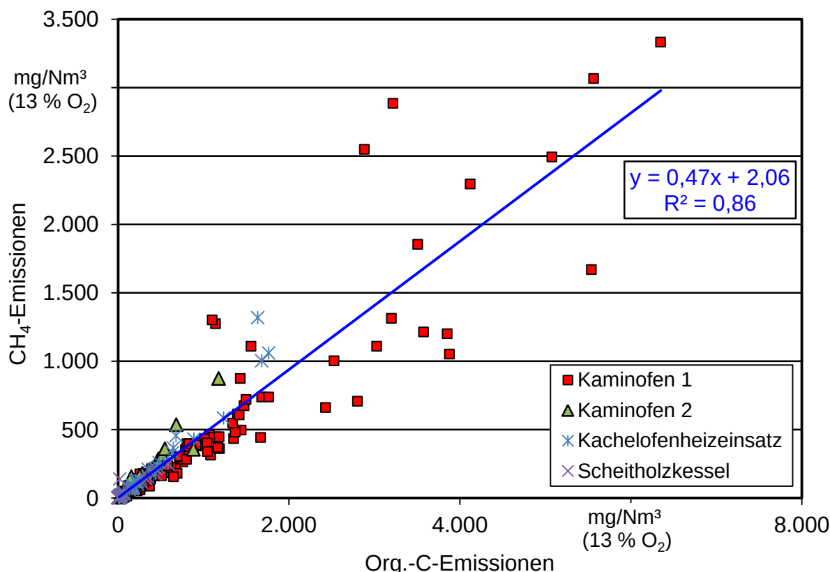
Abbildung 29: Anteil der Methanemissionen an den Kohlenwasserstoffemissionen, welche nicht kondensieren können. Auswertung von 227 Messungen an vier verschiedenen Feuerungen mit z. T. unterschiedlichen Brennstoffen
