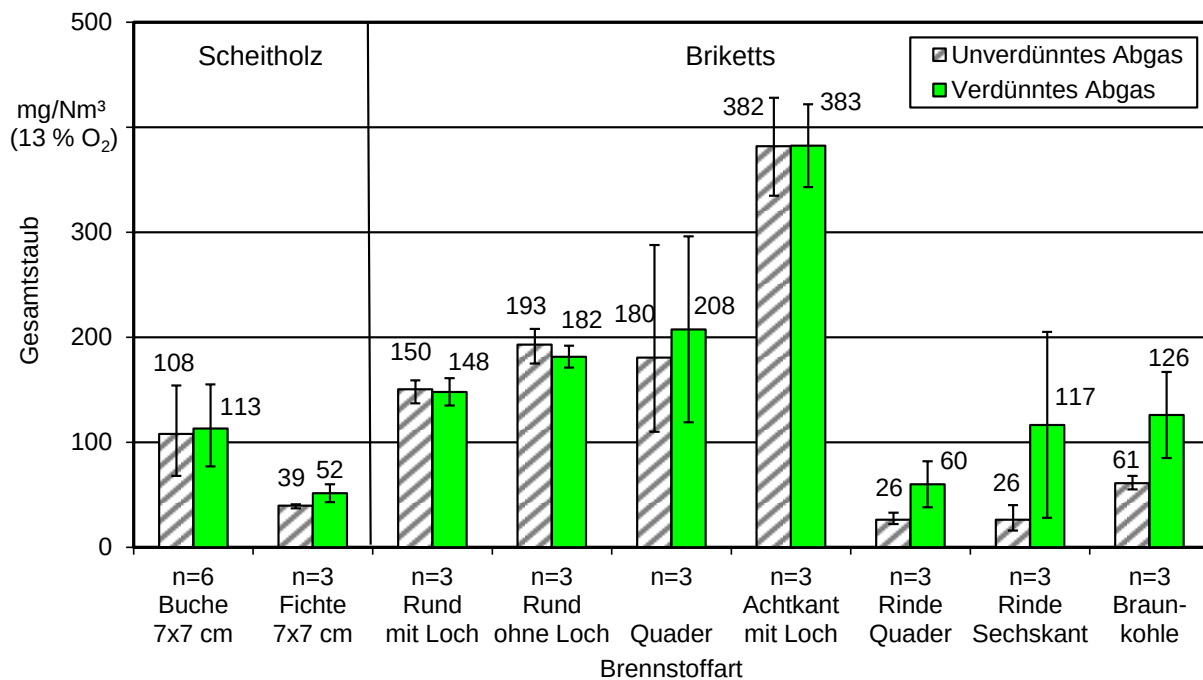
Abbildung 68: Vergleich der Staubemissionen von Scheitholz mit Holzbriketts, reinen Rindenbriketts und Braunkohlebriketts. Feuerung: Kaminofen 2 Fireplace Santa Fe, Nachlegemenge: ca. 1,6 kg (n = Anzahl der Messungen)
