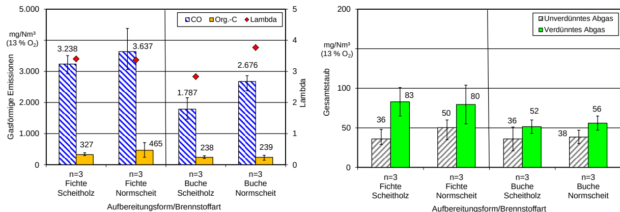
Abbildung 26: Vergleich des Emissionsverhaltens und der Reproduzierbarkeit der Messergebnisse unter Verwendung von Scheitholz und Normscheiten. Feuerung: Kaminofen 1 Buderus blueLine Nr. 12, Brennstoffe: Fichte und Buche ohne Rinde, Brennstoffmasse: 1,6 kg
