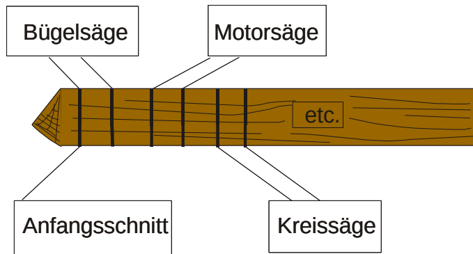
Abbildung 23: Schnittfolge für die Probenahme
