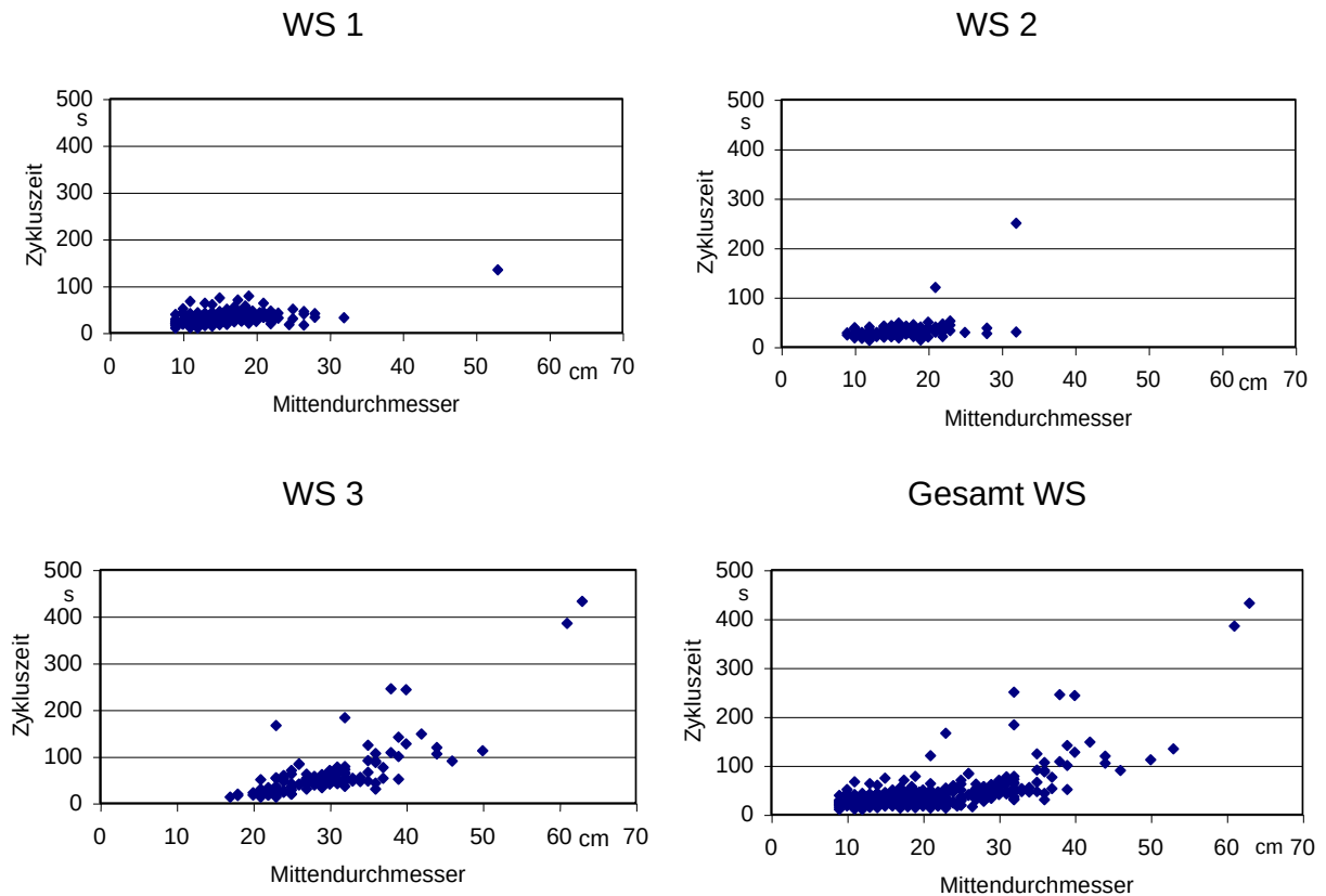
Abbildung 65: Zyklusdauer in Abhängigkeit vom Mittendurchmesser der Rundlinge bei den Waagerechtpalter(WS)-Studien
