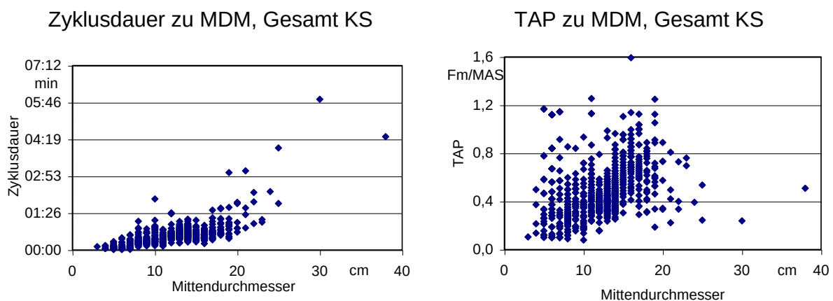
Abbildung 56: Zyklusdauer und technische Arbeitsproduktivität (TAP) in Abhängigkeit vom Mittendurchmesser (MDM) der Rundlinge (Werte aus allen Kleine-Senkrechtspalter(KS)-Studien)
