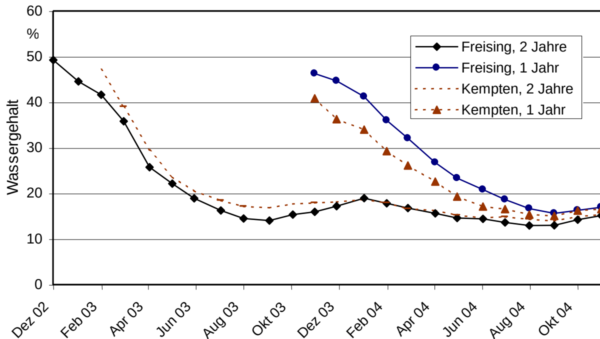
Abbildung 97: Vergleich des Trocknungsverlaufes von Buchenscheitholz an den Standorten Freising und Kempten. Lagerart: außen, abgedeckt, gespalten
