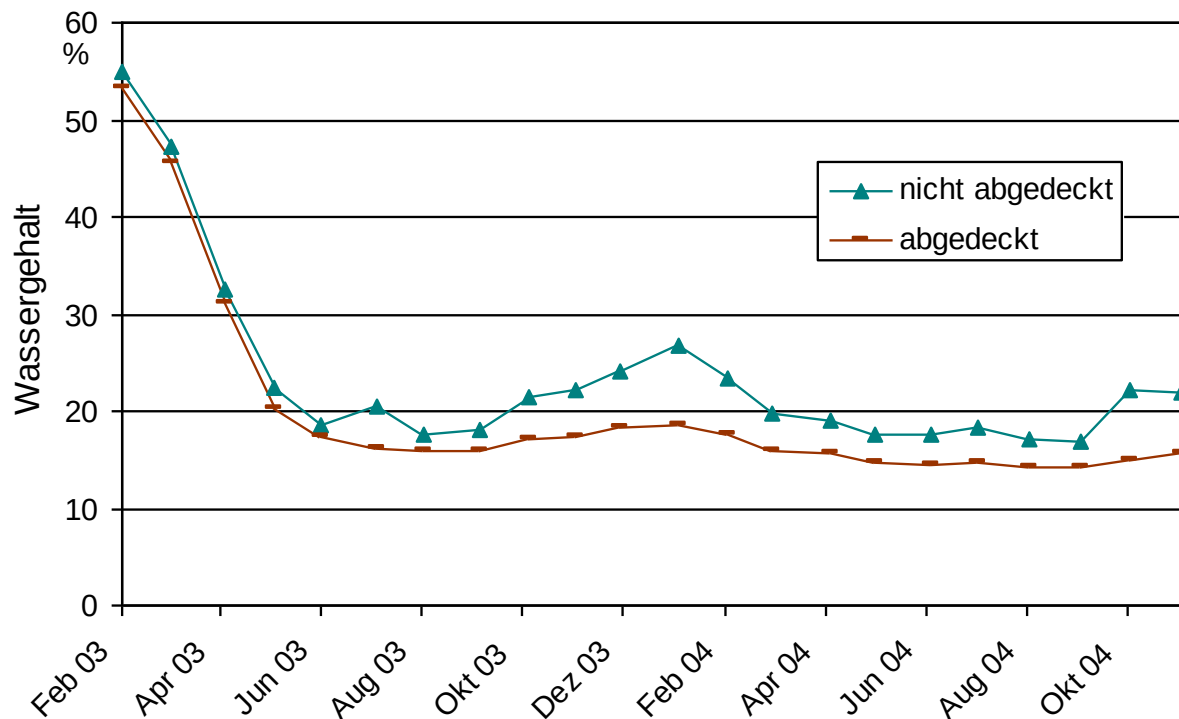
Abbildung 102: Vergleich der Lagerarten bei der Fichte am Standort Kempten
