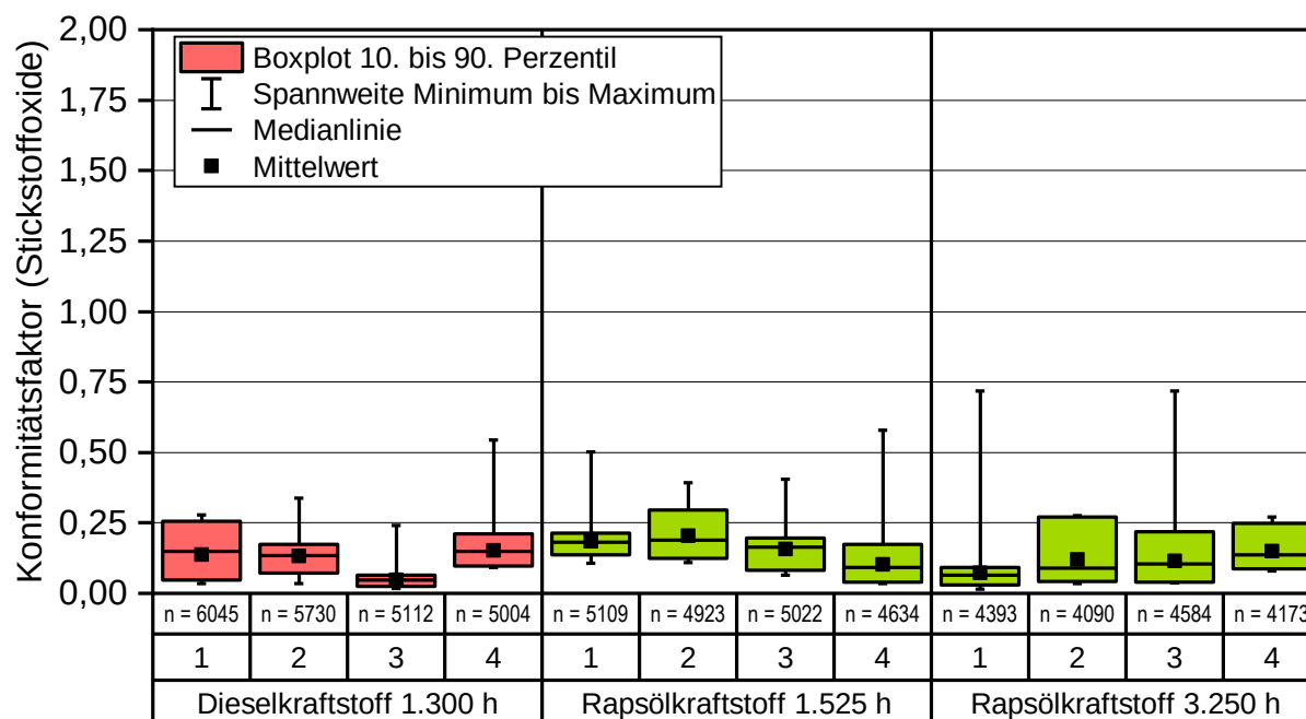
Abbildung 26: Häufigkeitsverteilung der resultierenden Konformitätsfaktoren für Stickstoffdioxid der Mittelungsfenster aus den Emissionsmessungen im realen Einsatz im Betrieb mit Diesel- und Rapsölmotorkraftstoff (n: Anzahl der Mittelungsfenster)
