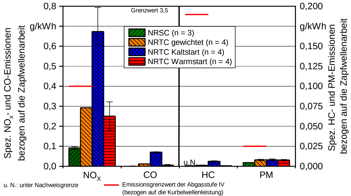
Abbildung 16: Mittelwerte und Spannweiten der spezifischen Emissionen von NO x , CO, HC und PM nach der Abgasnachbehandlung (AGN) des Traktors mit einem baugleichen Motor wie im Harvester John Deere 1470G und einer ECU-Konfiguration für Harvester im Betrieb mit Rapsölkraftstoff bei verschiedenen Prüfzyklen
