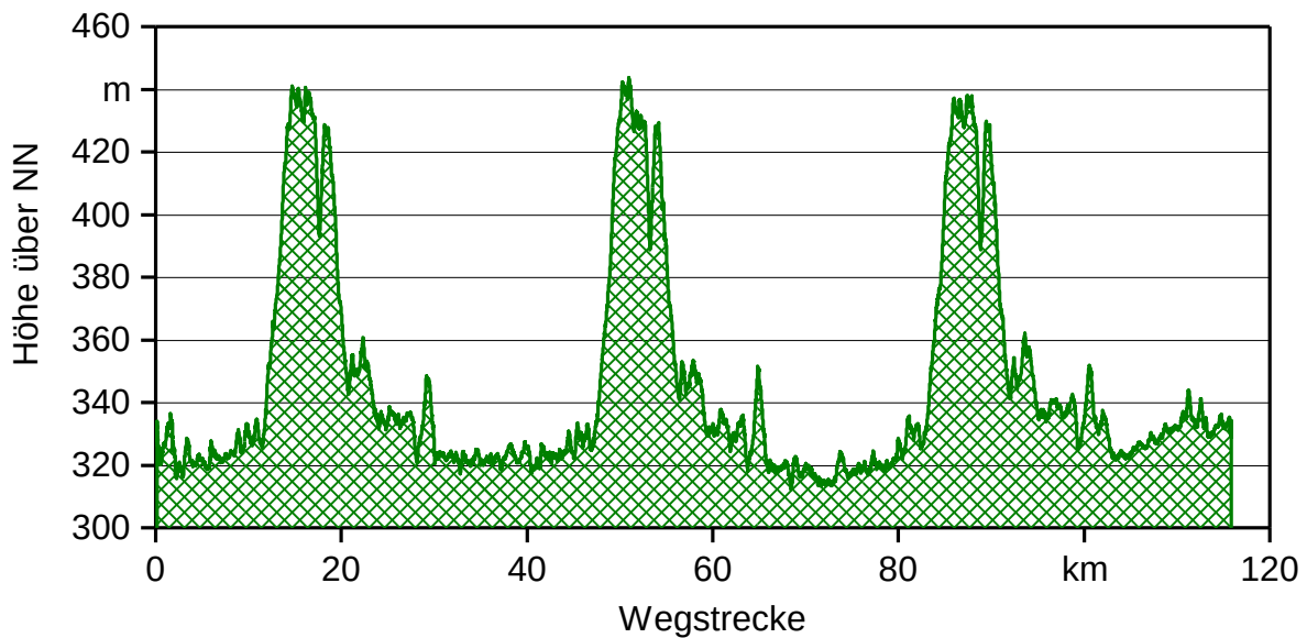
Abbildung 11: Höhenprofil der Teststrecke für Traktoren Version 2018
