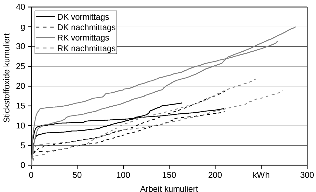
Abbildung 43: Kumulierte Stickstoffoxidmasse aufgetragen über der kumulierten Arbeit für Messungen mit Diesel- und Rapsölkraftstoff zu unterschiedlichen Tageszeiten
