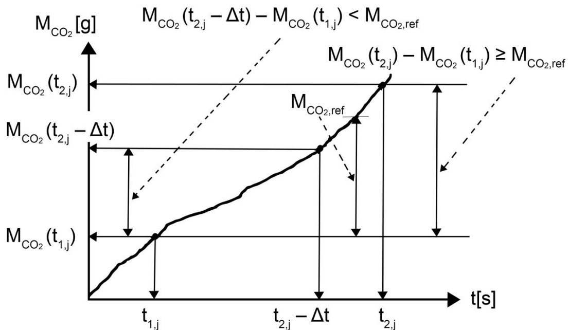
Abbildung 1: Festlegung von Mittelungsfenstern auf Grundlage der CO 2 -Masse nach der „Moving Averaging Window (MAW)“-Methode, eigene Darstellung nach [16]
