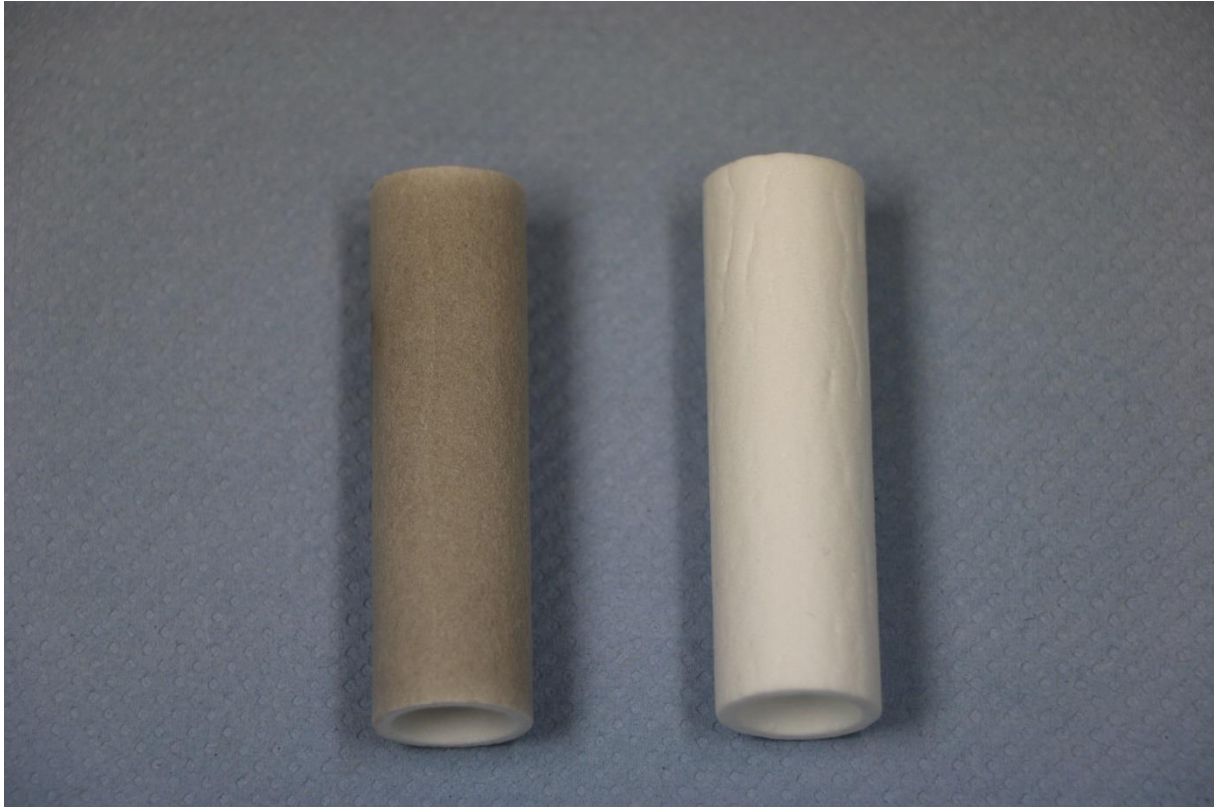
Abbildung 55: Abgasprobenfilter nach je einer Messfahrt im E10-Betrieb (links) und CNG-Betrieb (rechts)
