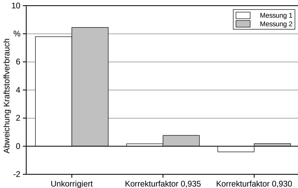
Abbildung 33: Abweichung des berechneten vom gemessenen Dieselkraftstoffverbrauch mit unterschiedlichen Korrekturfaktoren des Abgasmassenstroms
