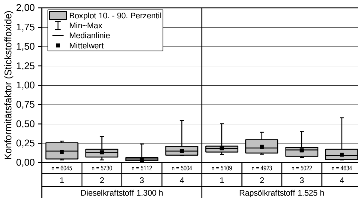
Abbildung 44: Boxplot-Darstellung der Verteilung der ermittelten Stickstoffoxid-Konformitätsfaktoren bei allen Fahrten gekürzt auf die sechsfache NRTC-Arbeit (144 kWh)
