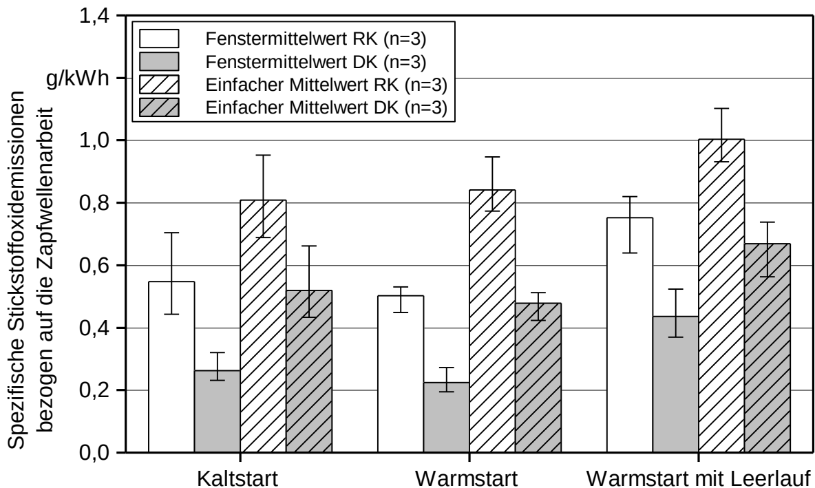
Abbildung 27: Vergleich der \text{NO}_x -Emissionsmittelwerte aller gültigen Fenster (Fenstermittelwert) mit dem Quotienten aus \text{NO}_x -Schadstoffmasse und gesamter verrichteter Arbeit (einfacher Mittelwert)
