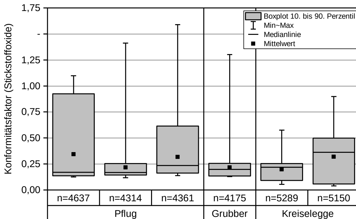
Abbildung 24: Stickstoffoxid-Konformitätsfaktoren aller Mittelwertfenster des Fendt 724 S4 im Betrieb mit Rapsölkraftstoff bei unterschiedlichen Arbeitsvorgängen
