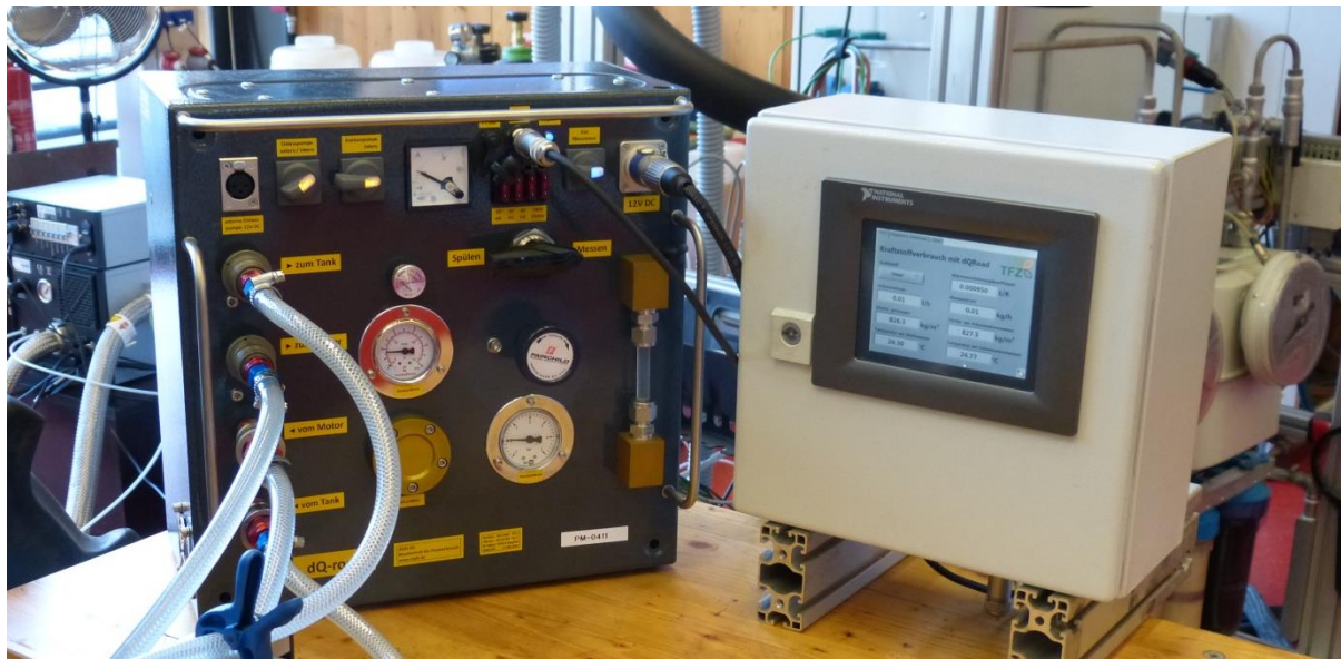
Abbildung 6: Kraftstoffverbrauchsmessgerät dQRoad (links) und Datenerfassungssystem (rechts)
