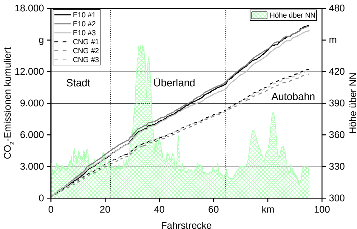
Abbildung 51: Kumulierte CO 2 -Emissionen über der Fahrstrecke, Höhenprofil und Einteilung in Stadt-, Überland- und Autobahnabschnitte
