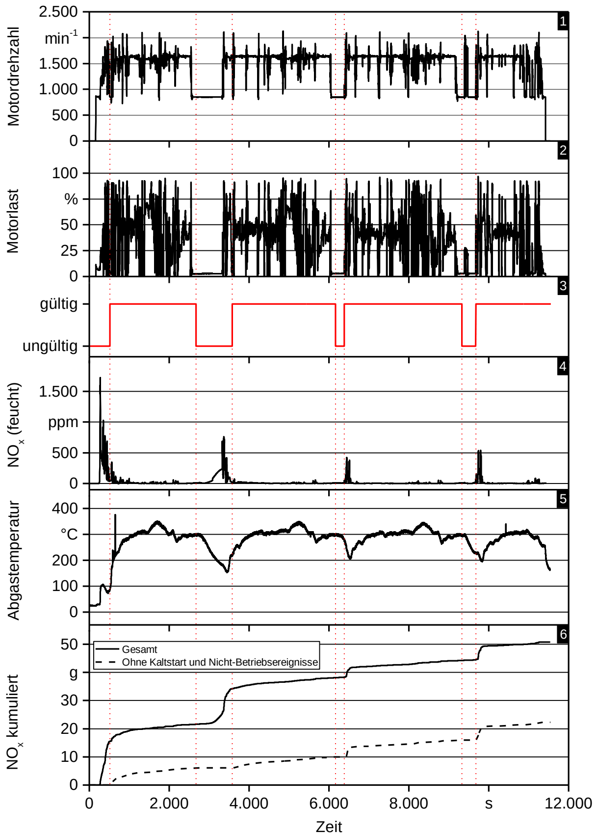
Abbildung 37: Motordrehzahl und -last, Stickstoffoxidemissionen, Abgastemperatur und Gültigkeitsbereiche einer Messfahrt mit Kaltstart und Nicht-Betriebsereignissen
