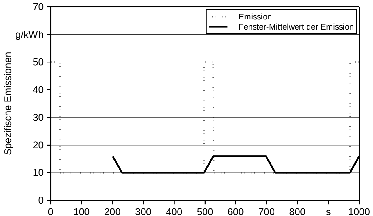
Abbildung 28: Fiktiver Emissionsverlauf und Mittelwert der Emission je Fenster mit einer Fensterdauer von 200s
