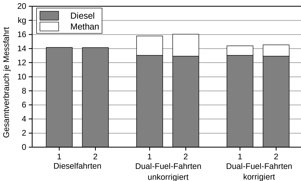
Abbildung 35: Gesamt-Kraftstoffverbräuche des Traktors bei zwei Diesel- und zwei Dual-Fuel-Messfahrten mit unkorrigiertem und korrigiertem Methanverbrauch
