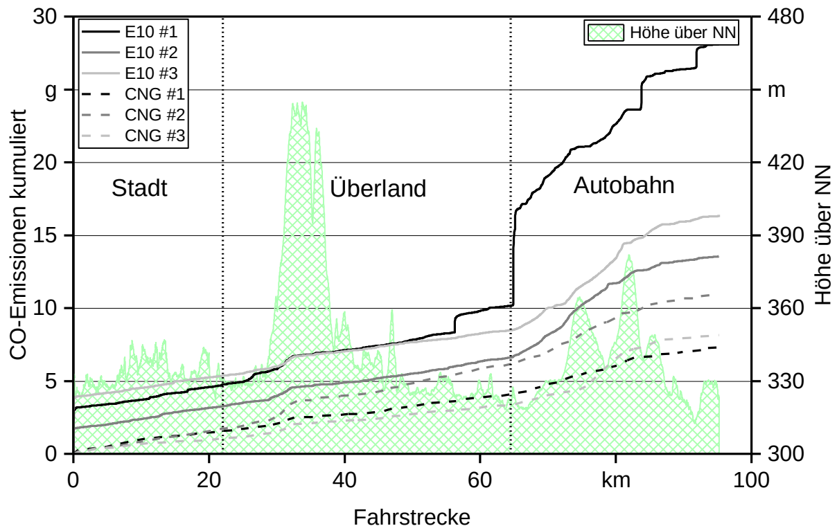
Abbildung 52: Kumulierte CO-Emissionen über der Fahrstrecke, Höhenprofil und Einteilung in Stadt-, Überland- und Autobahnabschnitte
