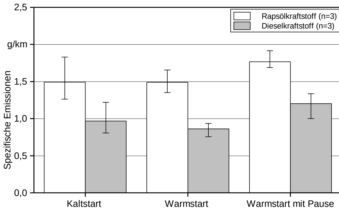
Abbildung 29: Stickstoffoxidemissionen des untersuchten und für Dieselmotorkraftstoff optimierten Traktors bei Straßenfahrten mit Rapsöl- und Dieselmotorkraftstoff bezogen auf die Fahrstrecke (Etappenwert)
