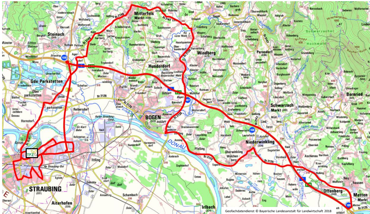
Abbildung 12: Teststrecke für PKW Version 2018
