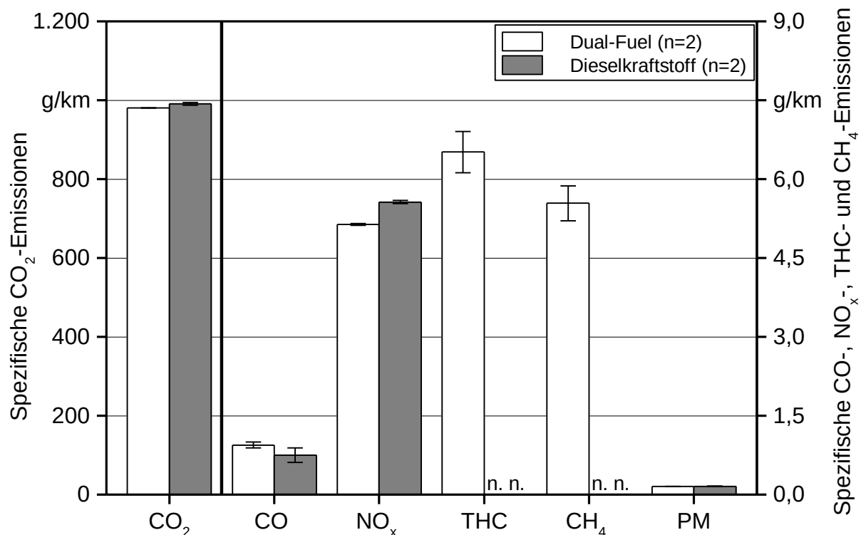
Abbildung 32: Emissionen des Traktors Valtra 101 H Dual-Fuel bei RDE-Messungen auf der Traktor-Teststrecke
