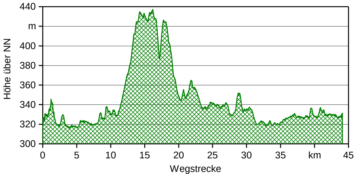
Abbildung 9: Höhenprofil der Teststrecke für Traktoren Version 2016
