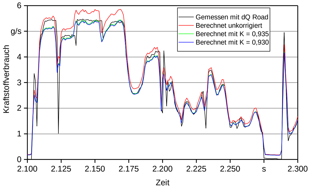
Abbildung 34: Ausschnitt des Verlaufs des Dieselkraftstoffverbrauchs gemessen mit dQRoad und berechnet nach der Kohlenstoffbilanz-Methode mit verschiedenen Korrekturfaktoren
