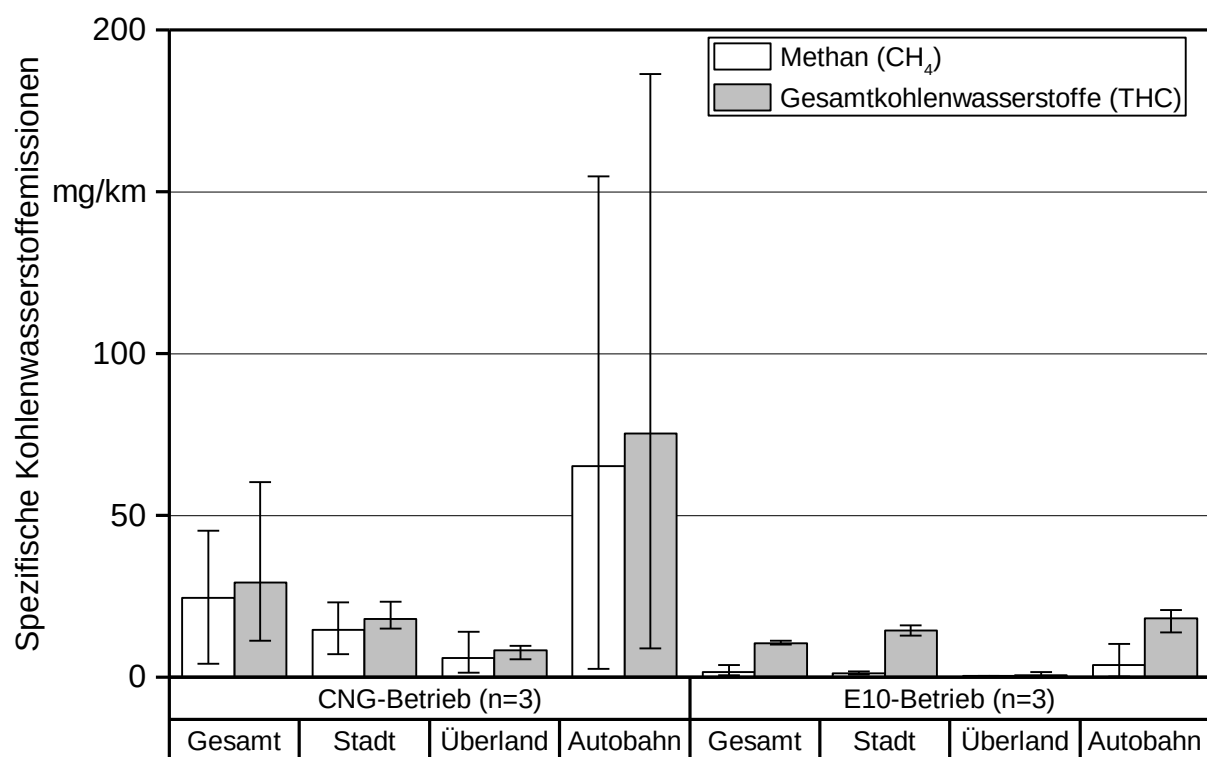
Abbildung 54: Methan- und Gesamtkohlenwasserstoffemissionen des Audi A3 g-tron auf der gesamten Teststrecke und aufgeteilt in Stadt-, Überland- und Autobahnanteil
