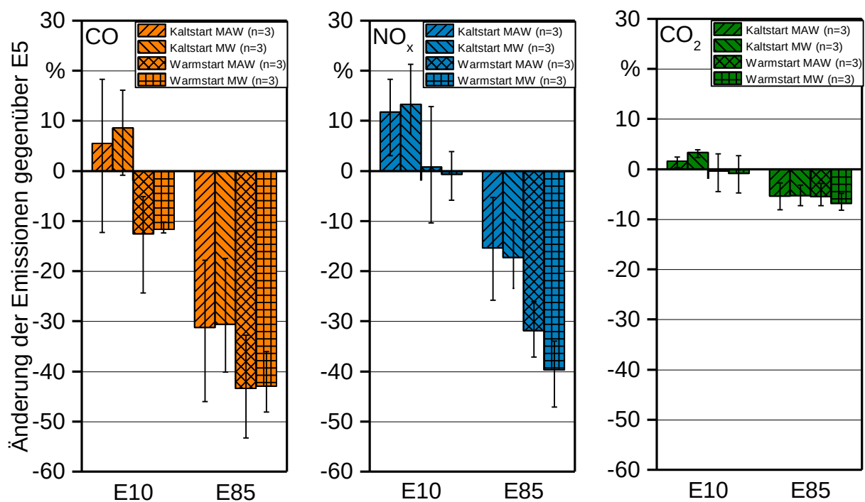
Abbildung 47: Änderung der Kohlenstoffmonoxid-, Stickstoffoxid- und Kohlenstoffdioxidemissionen beim Einsatz von E10 bzw. E85 gegenüber E5 bei den durchgeführten Realfahrtmessungen [22]
