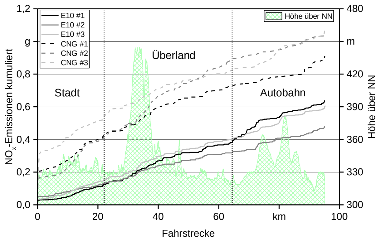
Abbildung 53: Kumulierte \text{NO}_x -Emissionen über der Fahrstrecke, Höhenprofil und Einteilung in Stadt-, Überland- und Autobahnabschnitte
