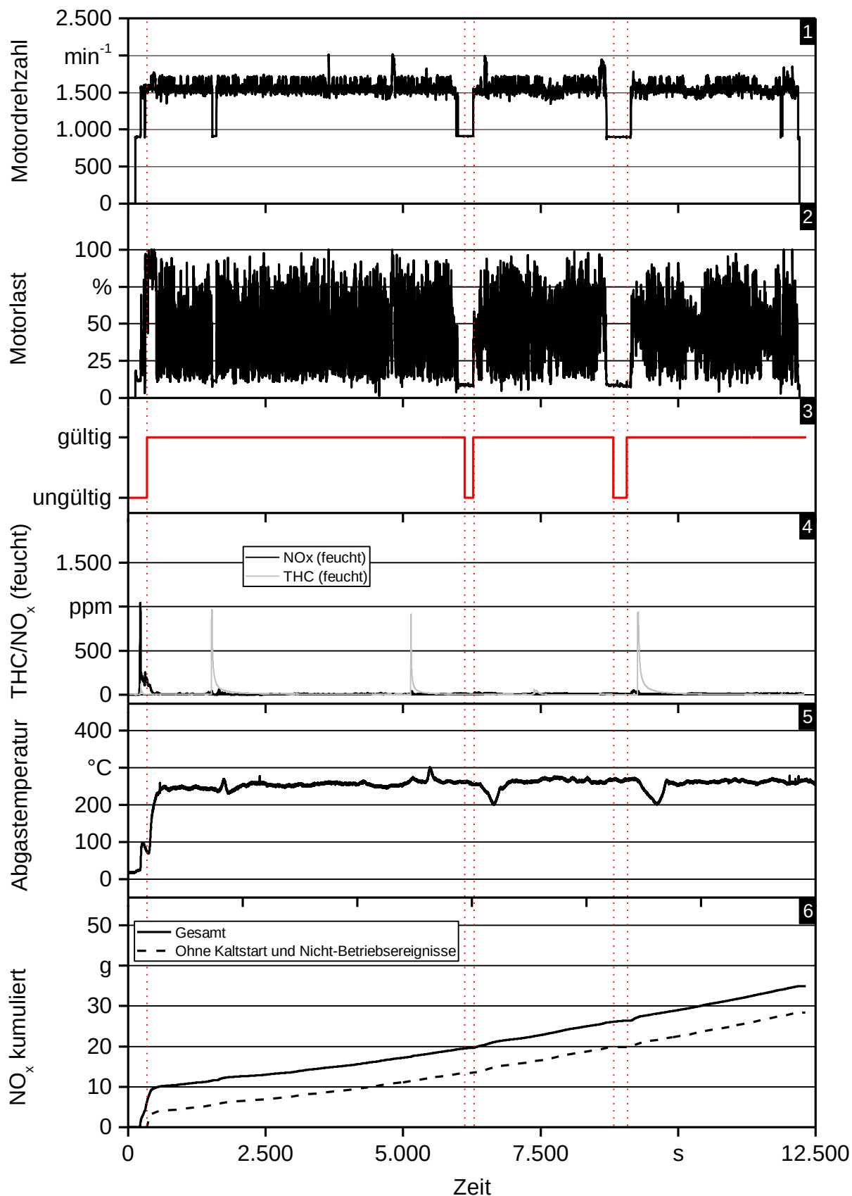
Abbildung 42: Motordrehzahl und -last, NO x - und THC-Emissionen, Abgastemperatur und Gültigkeitsbereiche einer Messfahrt mit Kaltstart und Nicht-Betriebsereignissen
