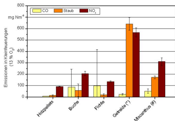
Abb. 2: Bei der Verbrennung gemessene Emissionen an CO 2 , Staub und NO x verschiedener Brennstoffe (*Ganzpflanzen-Pellets; #gehäckselte)
