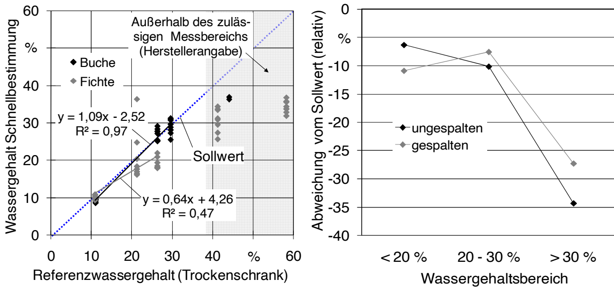
Abbildung 24: Absolute Abweichung bei der Feuchte-Schnellbestimmung zum Referenzwassergehalt in Abhängigkeit der Holzart und Wassergehalt (links) bzw. relative Abweichung zum Sollwert in Abhängigkeit von Holzvorbereitung und Wassergehalt (rechts); Messgerät Gann, Hydromette HT 65 mit Elektrode M 18
